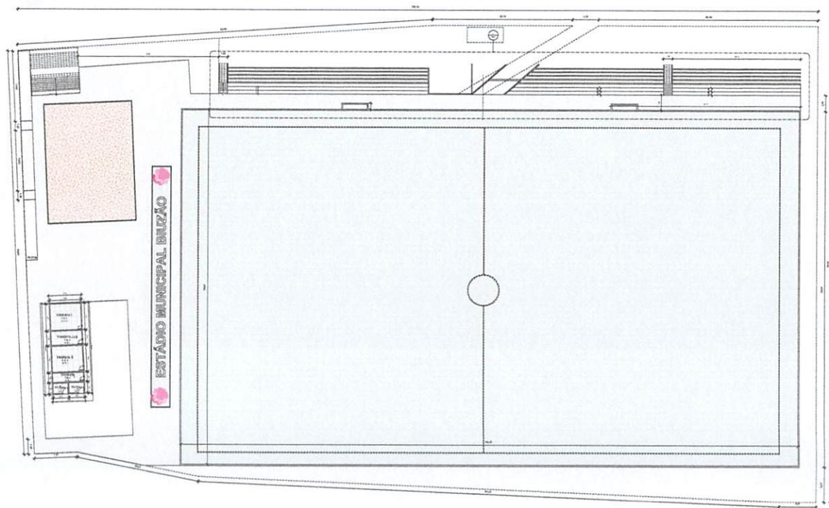
1 PLANTA BAIXA - TERREO Escala: 1:200
